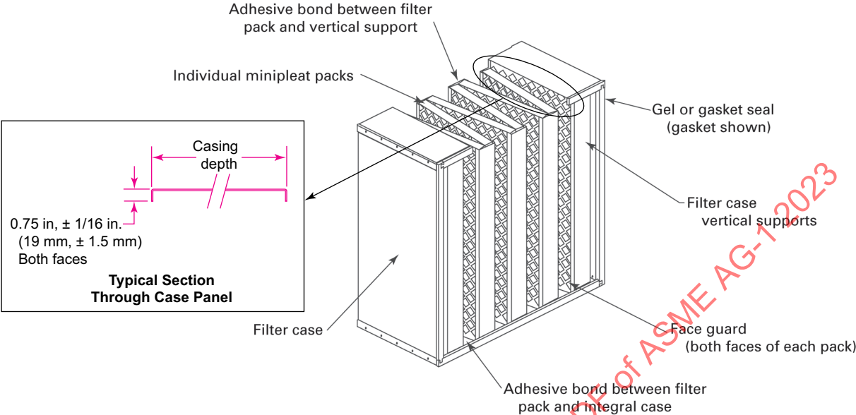
Figure FC-4110-3 Type B Mini Pleat Filter
