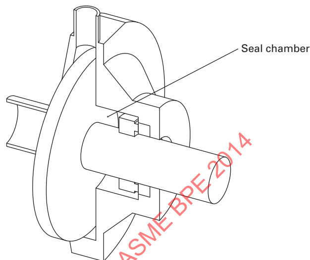
Fig. SG-2.3.2.4-2 Flush Plan 02
