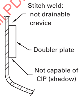
(d) Poor Design (Not Accepted)
