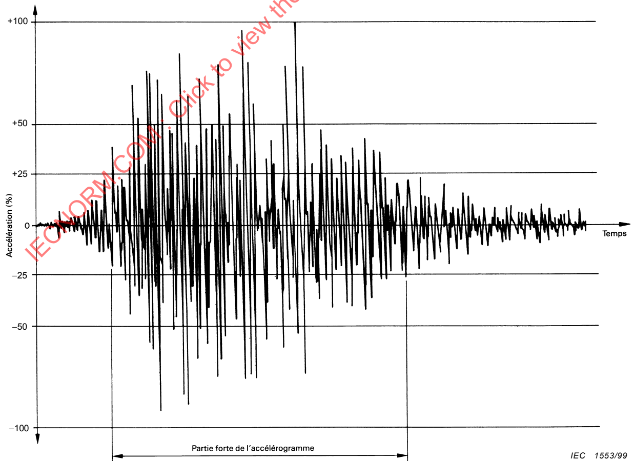
Figure 4 – Accélérogramme typique
