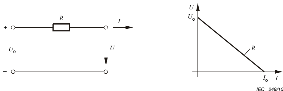
Figure C.1a – Caractéristiques linéaires
