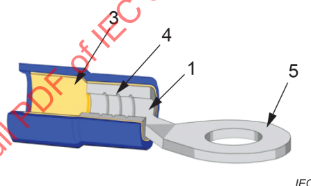
b) version avec fût en laiton pour manchon isolant
