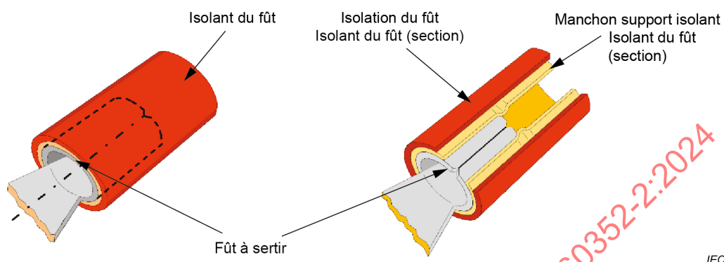
Figure 10 – Fût à sertir pré-isolé
