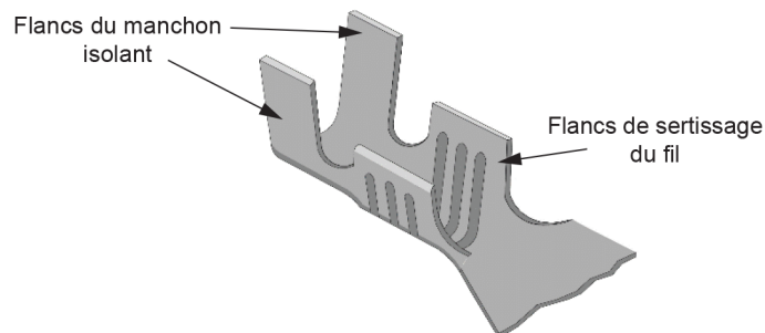
Figure 8 – Fût ouvert
