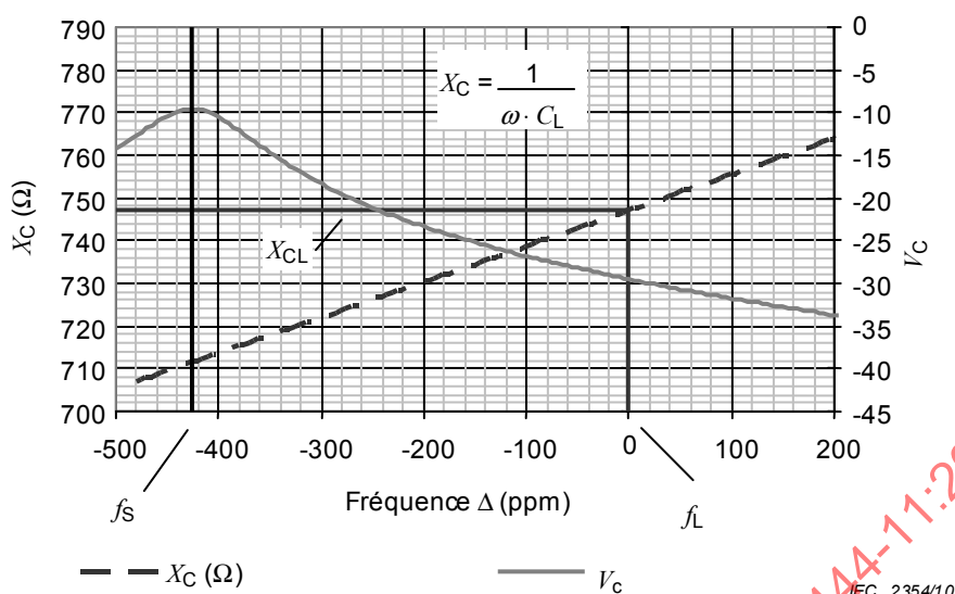
Figure 2 – X_C en fonction de la fréquence (ligne continue) au voisinage de f_L
