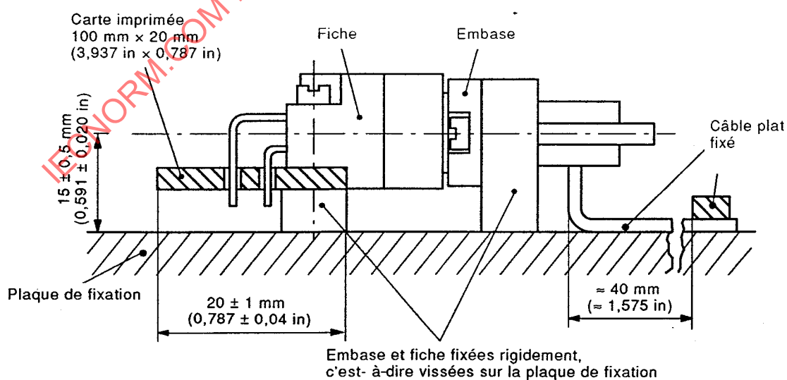
Figure 39 – Montage relatif à des connecteurs munis d'un câble plat (déplacement d'isolant)
