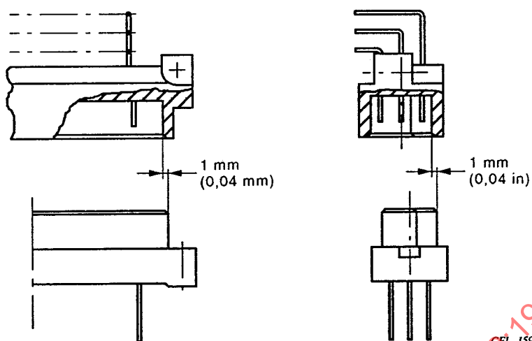
Figure 3 – Enfichage perpendiculaire
