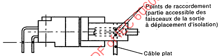
Figure 35 – Déplacement d'isolant
