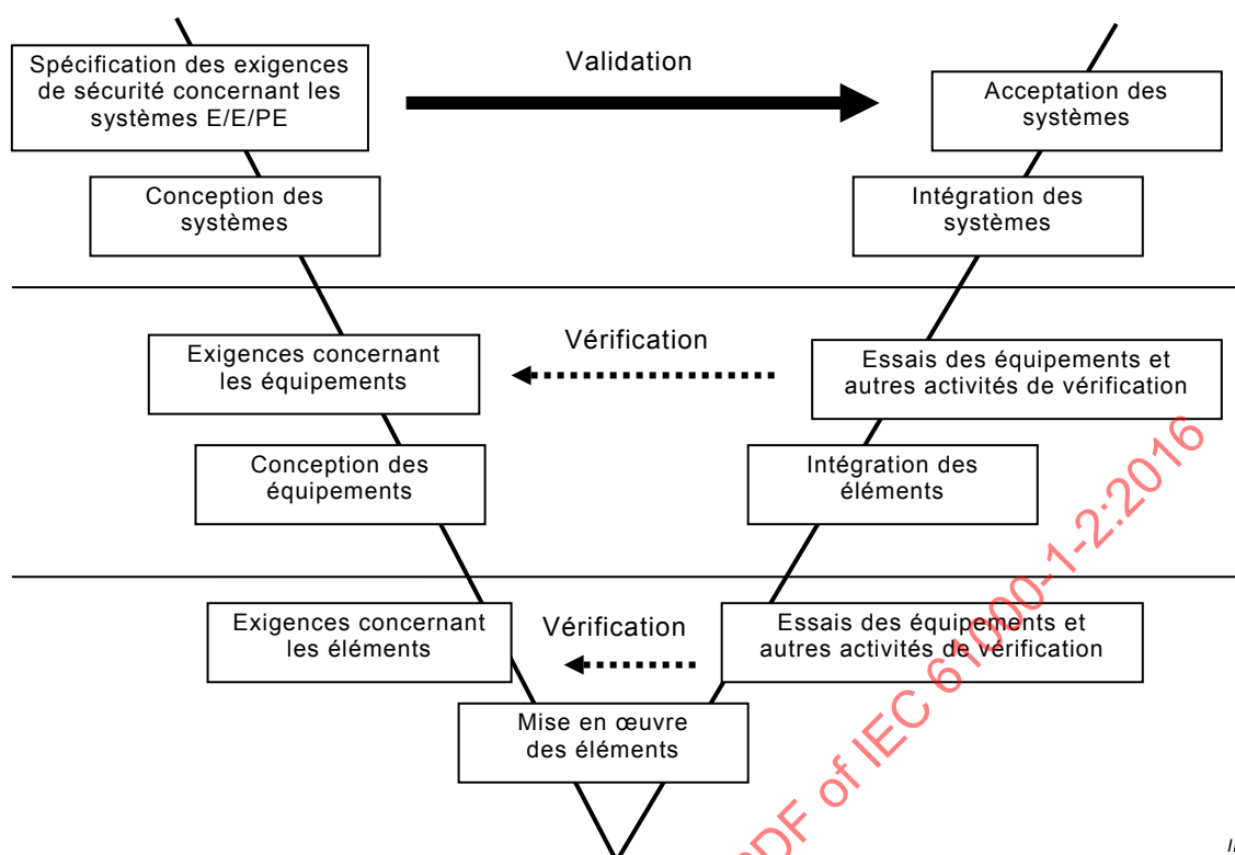
Figure 4 – Exemple de représentation en V des cycles de vie démontrant le rôle de la validation et de la vérification pour les performances de sécurité fonctionnelle par rapport aux perturbations électromagnétiques
