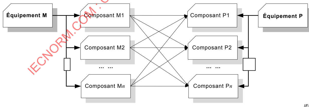
Figure 3 – CEM entre un équipement M et un équipement P
