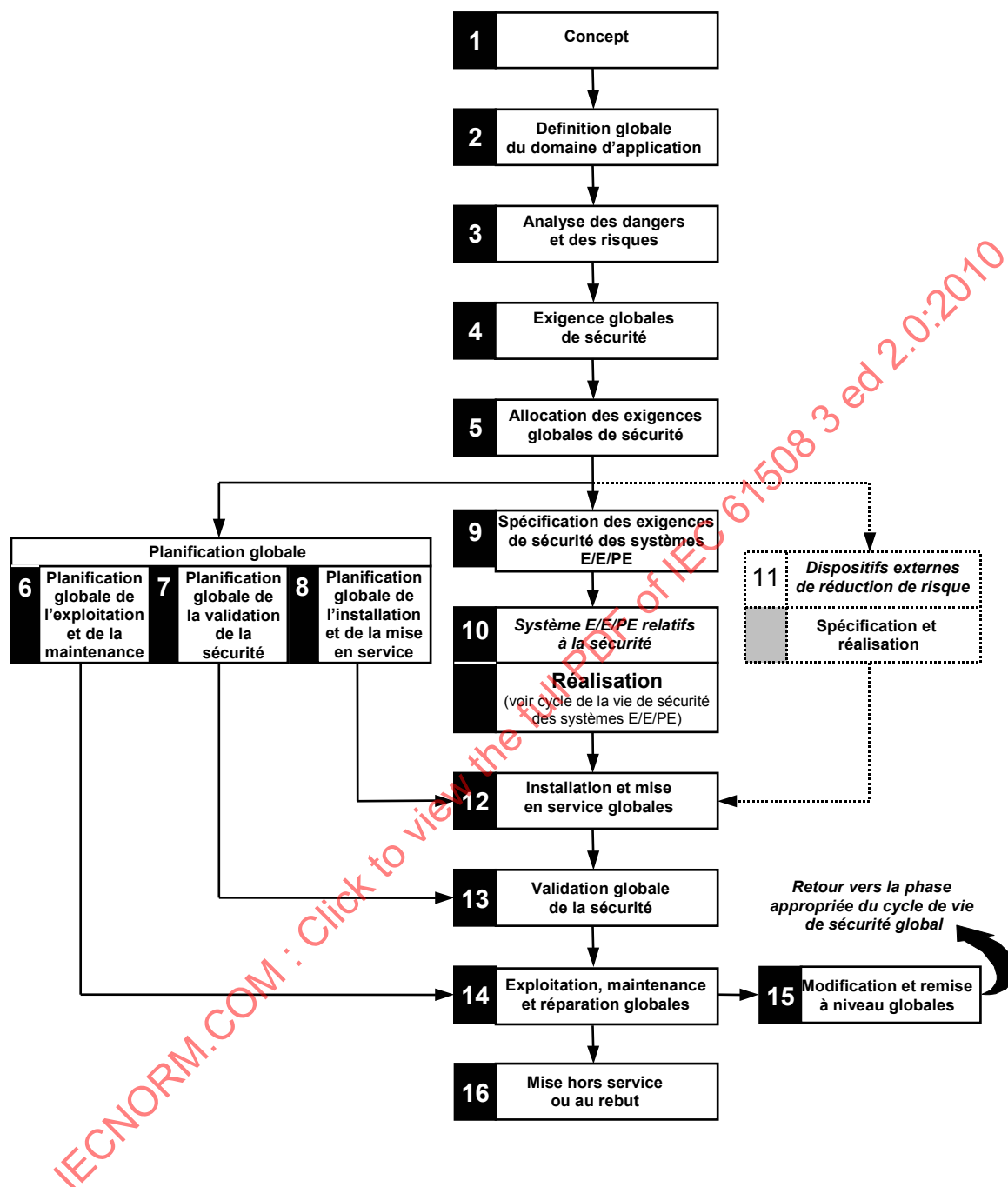
Figure 2 – Cycle de vie de sécurité global
