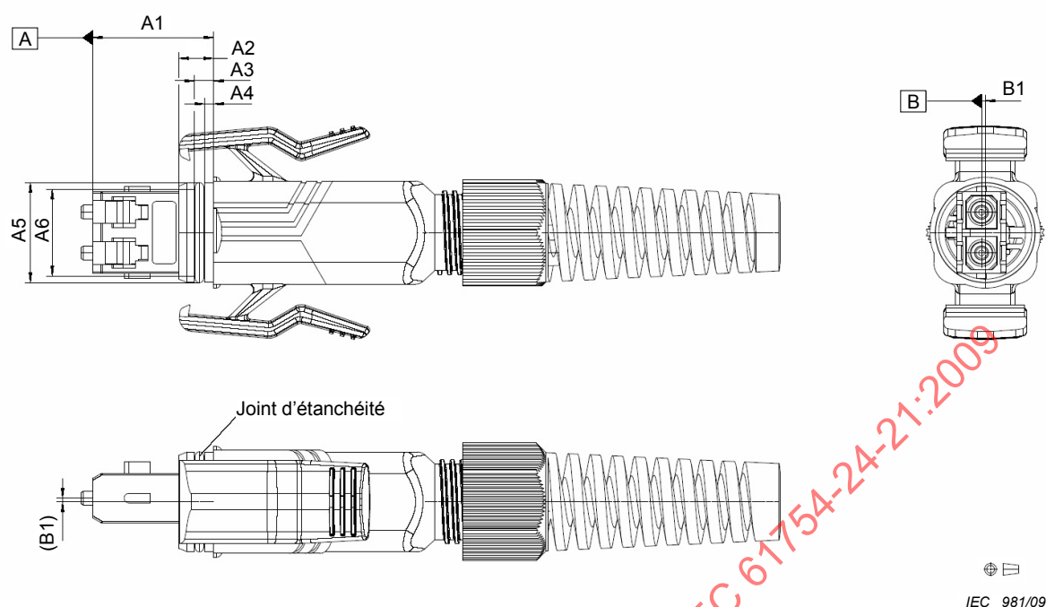
Figure 1 – Fiche (mâle)
