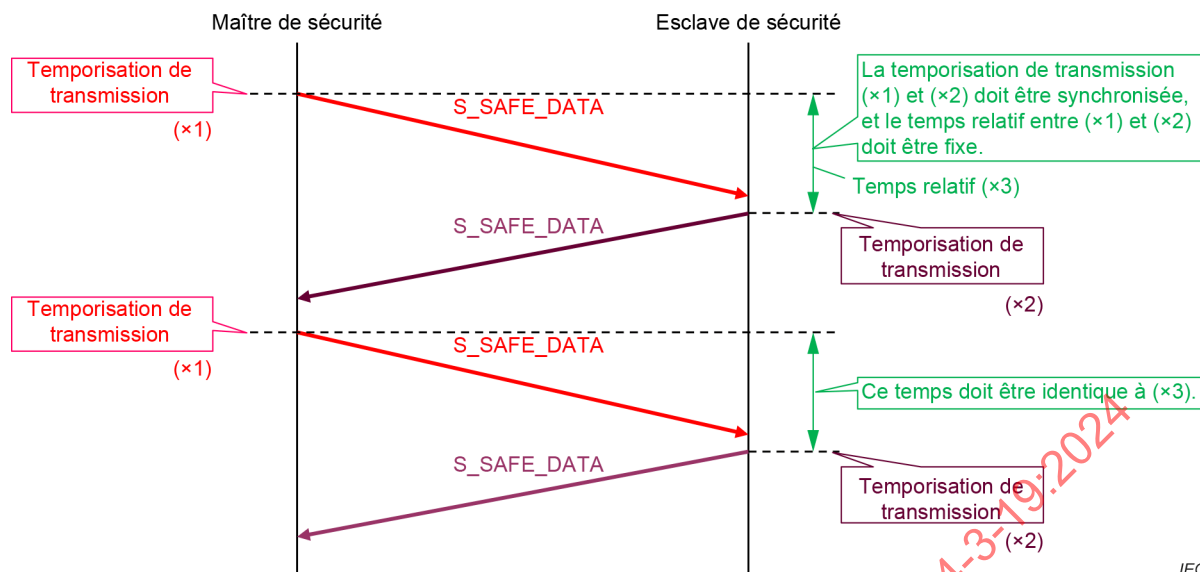
Figure 6 – Synchronisation de la temporisation de transmission
