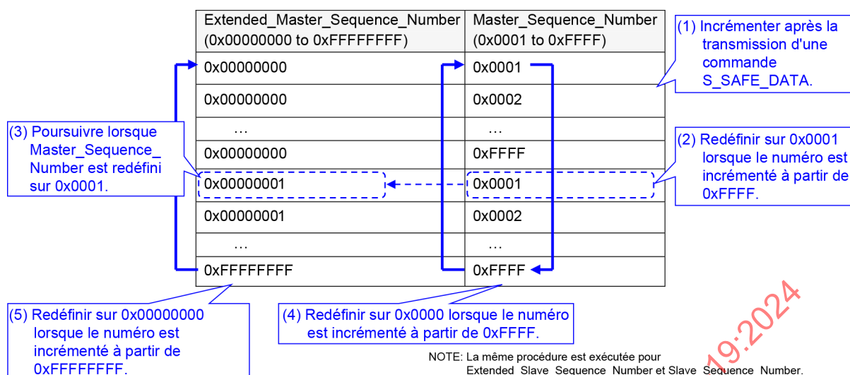
Figure 4 – Procédure d'incrémentation du numéro de séquence
