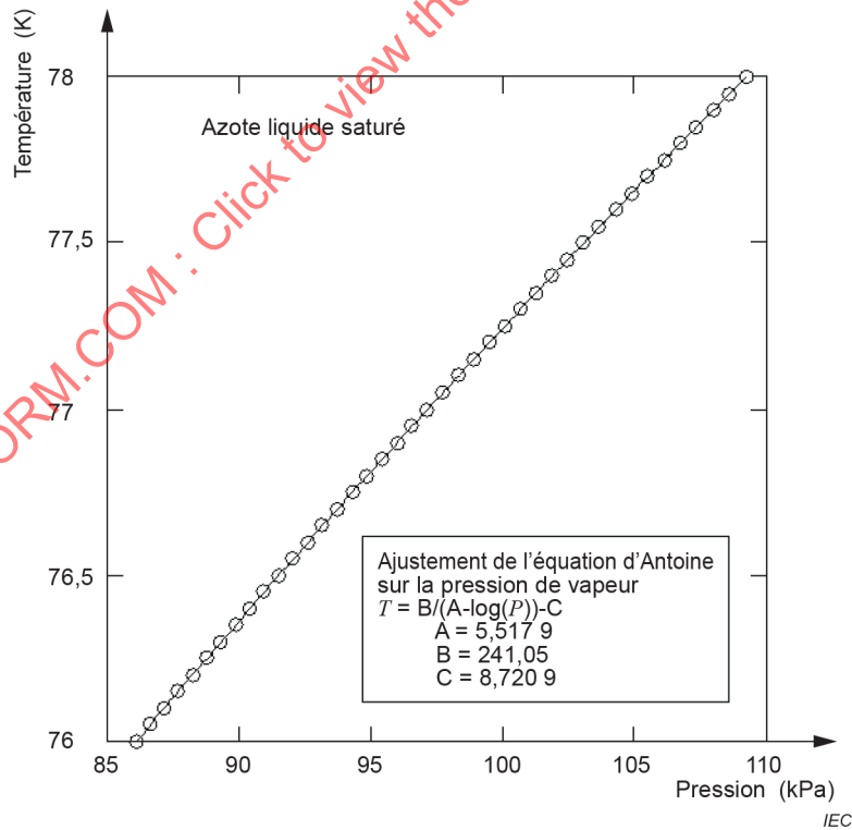
Figure A.3 – Dépendance de la température d'ébullition de l'azote liquide vis-à-vis de la pression
