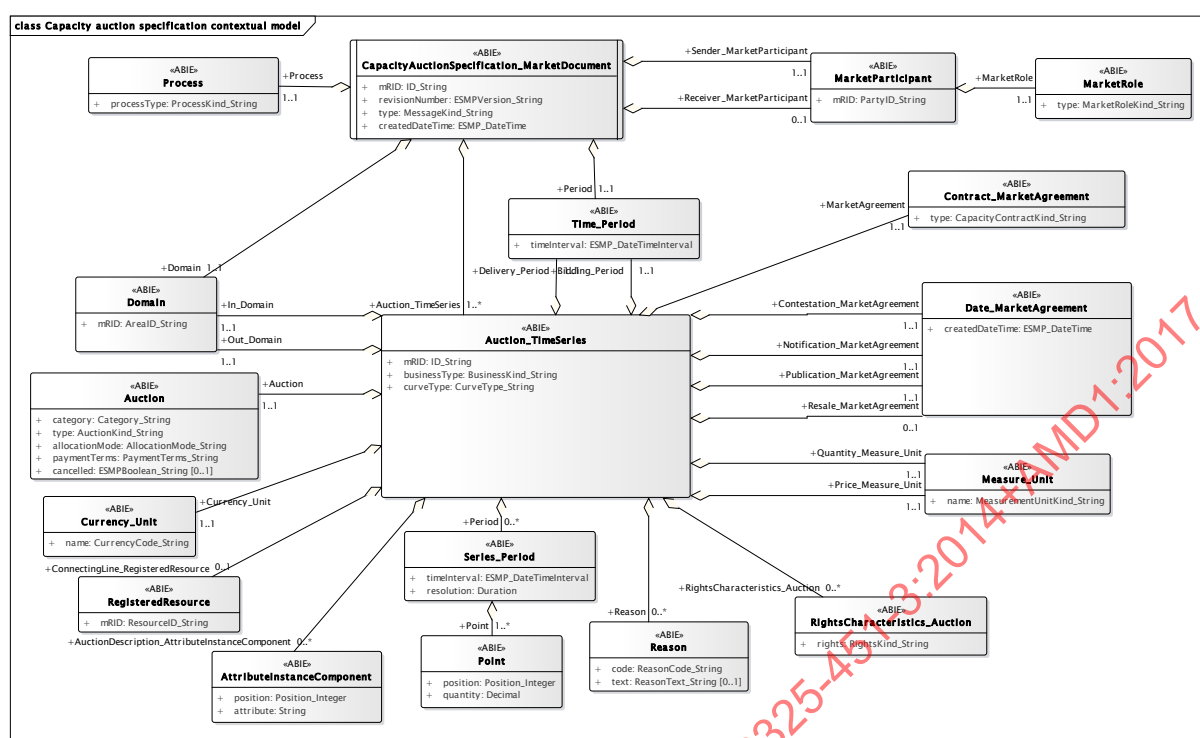
Figure 11 – Modèle contextuel de spécification de vente aux enchères de capacité
