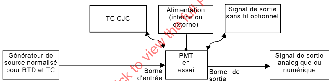
Figure 1 – Exemple schématique de configuration d'essai pour transmetteurs de mesure de température
