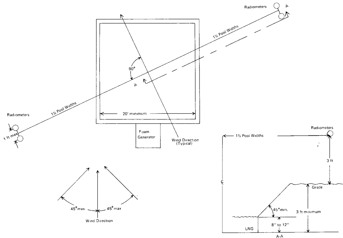
Figure A-1-10.5(d) Test Pit.
