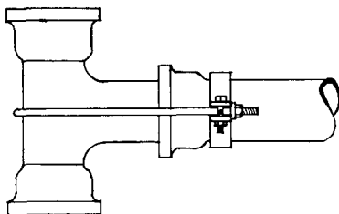
FIG. 96-10. TEE ANCHOR
