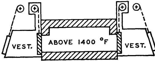
TYPE I
